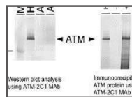
ATM
