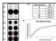
TRF-2
