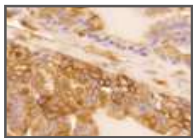
alpha-Tubulin
