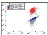
HIF-1-alpha
